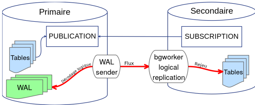
Figure 2: Schéma du fonctionnement de la répliation logique
